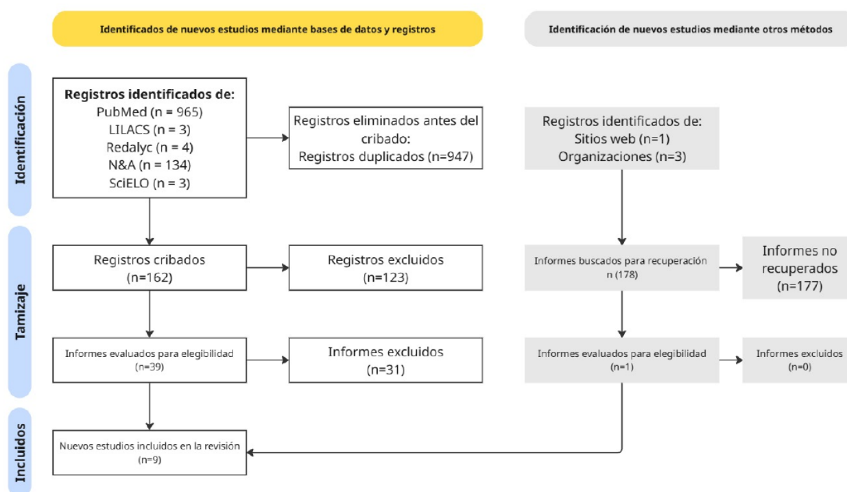
Figura 1. Flujograma PRISMA-ScR.
